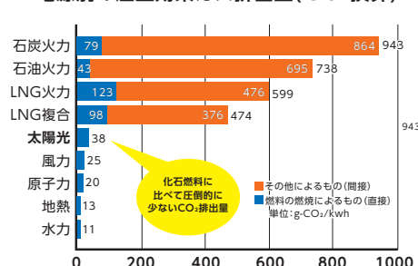
電源別の温室効果ガス排出量(CO 2 換算)
