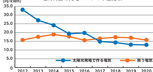
電気料金と発電コストの単価比較
